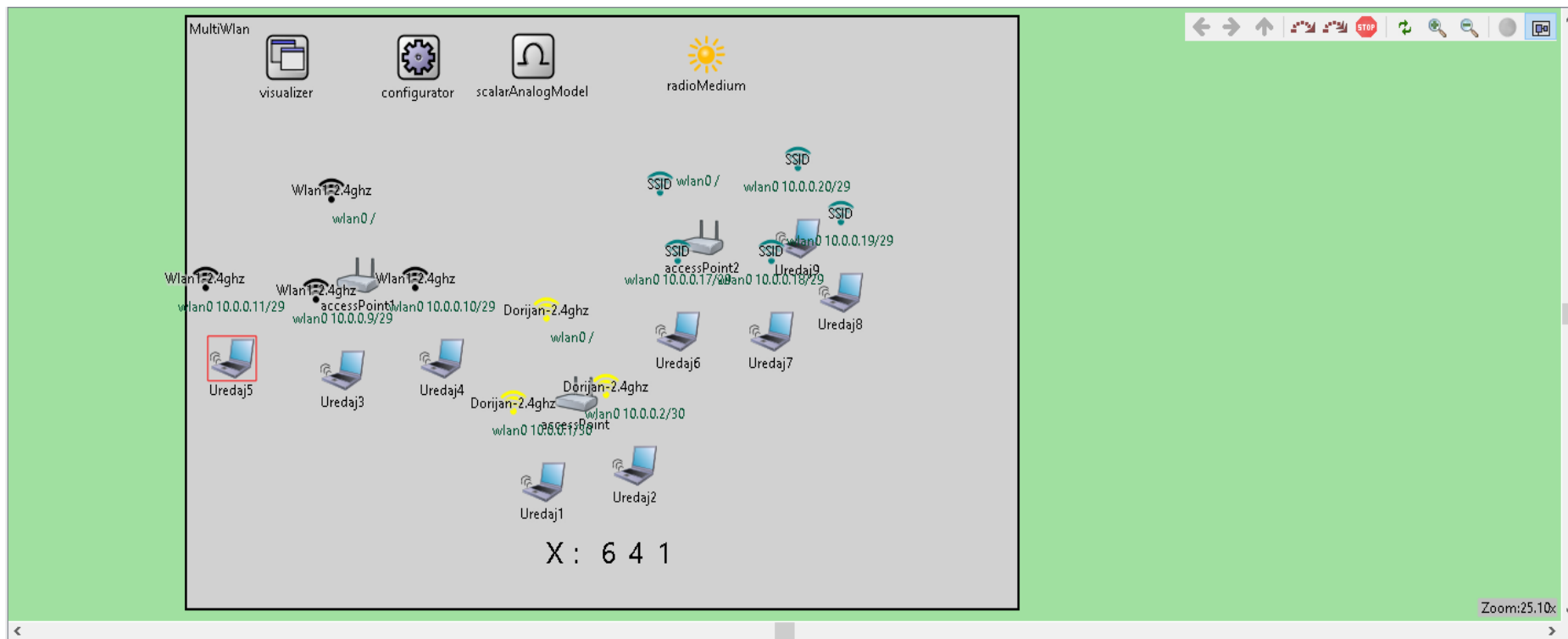
Slika 10. Simulacija međusobne interferencije mreža Wlan1 i Dorijan
